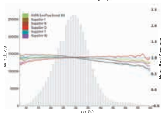
カバレッジの均一性
